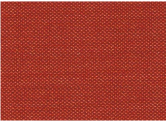
S-3 6788
