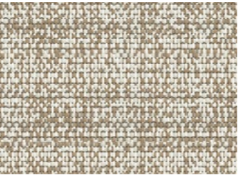
S-2 6733
