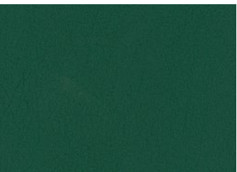
S-3 3122
