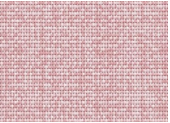
S-2 6741
