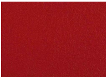
S-3 3116
